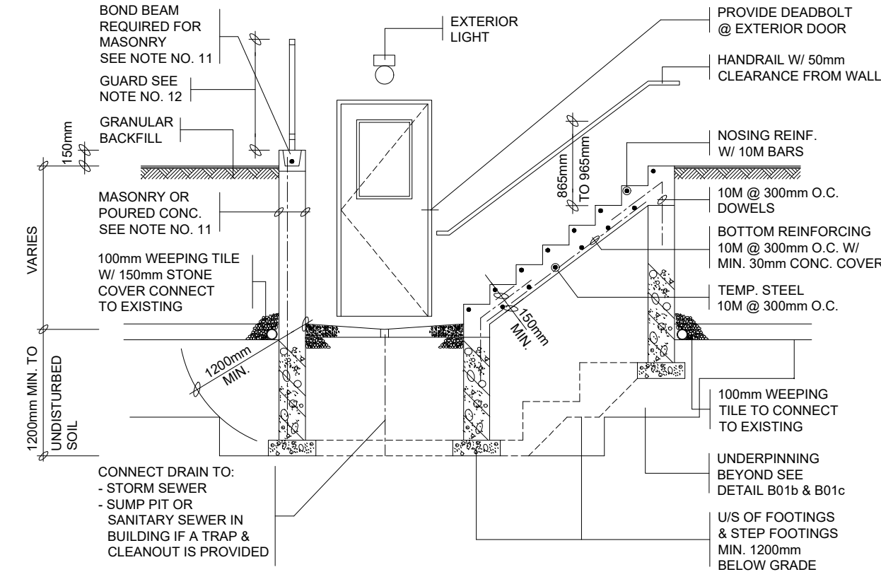
SECTION 'A'
