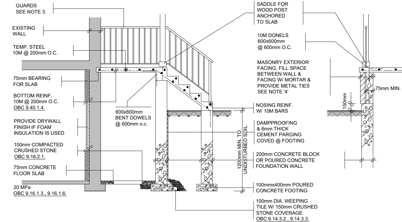
SECTION 'A'
